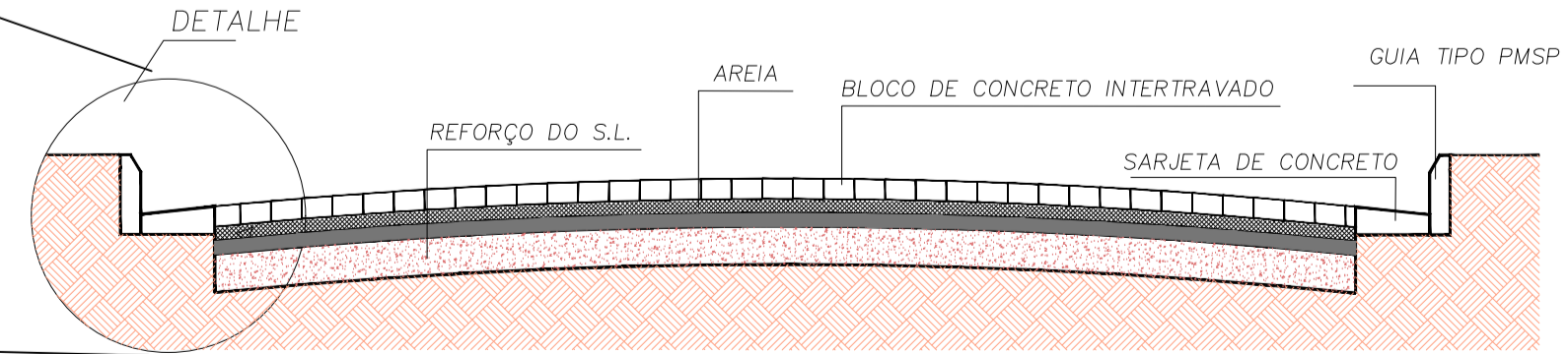
PEFIL TRANSVERSAL sem escala
