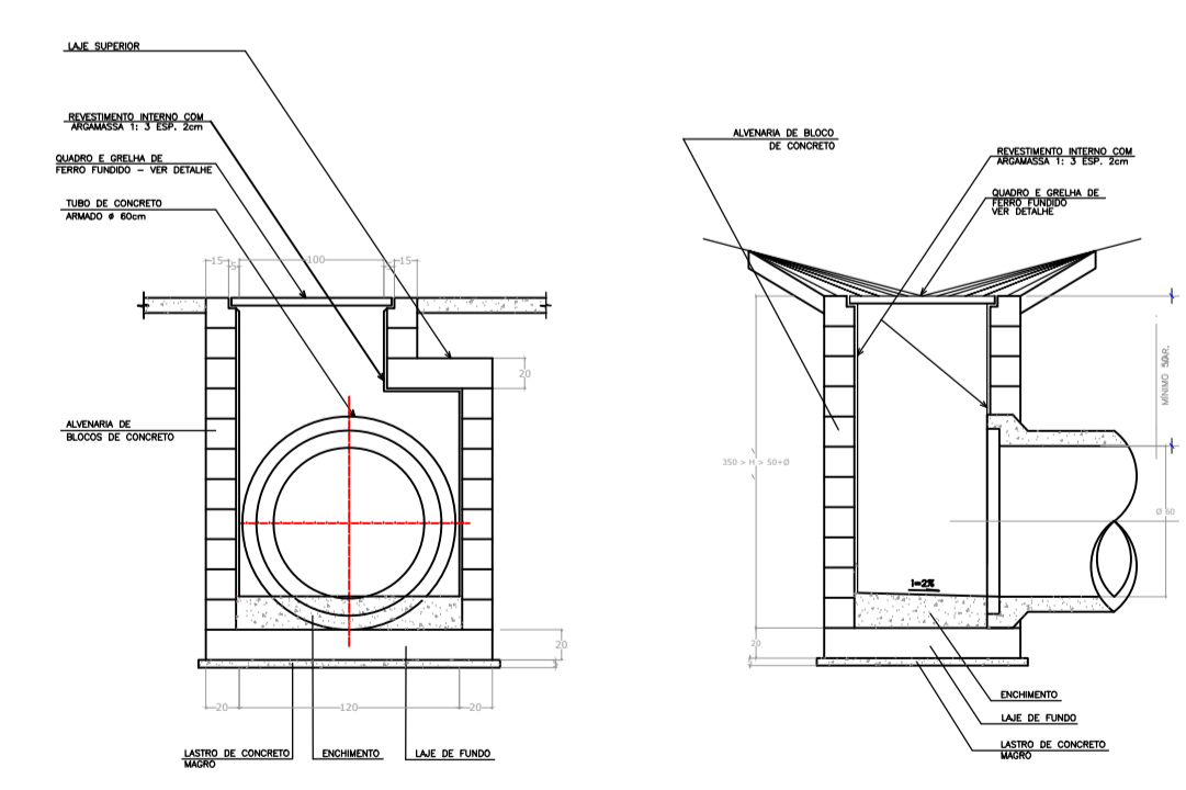
CORTE A DETALHAMENTO CAIXA COLETORA S/ ESC.
