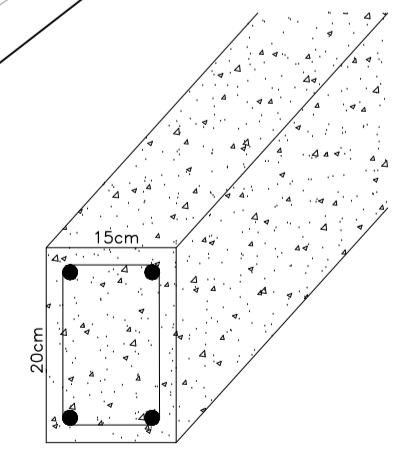
DETALHE VIGA DE TRAVAMENTO s/ esc.
